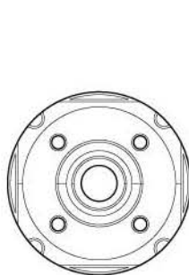
デフケース GB1 ×2 Differential gear case Differentialgehäuse Carter de différentiel
