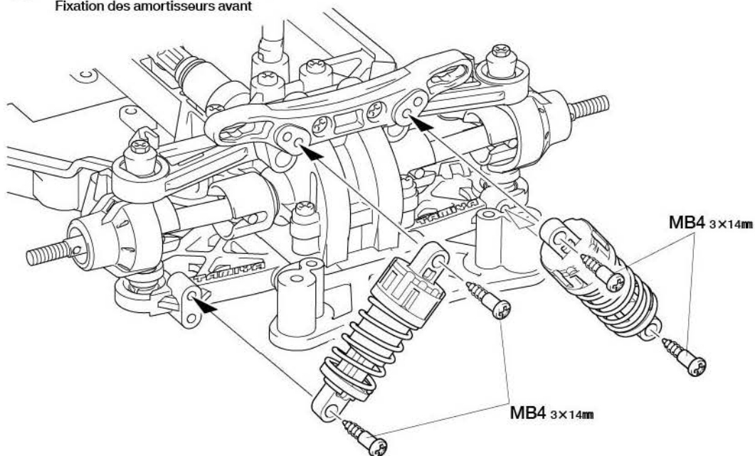
3×14mm段付タッピングビス Step screw Paßschraube Vis décollée
